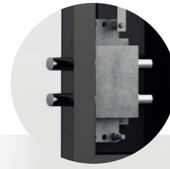
Due deviatori doppi a slitta inferiori
