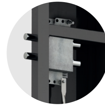
Due deviatori doppi a slitta superiori
