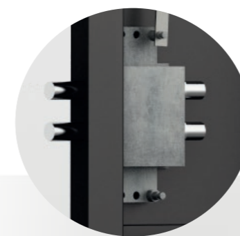
Deviatore doppio a slitta inferiore
